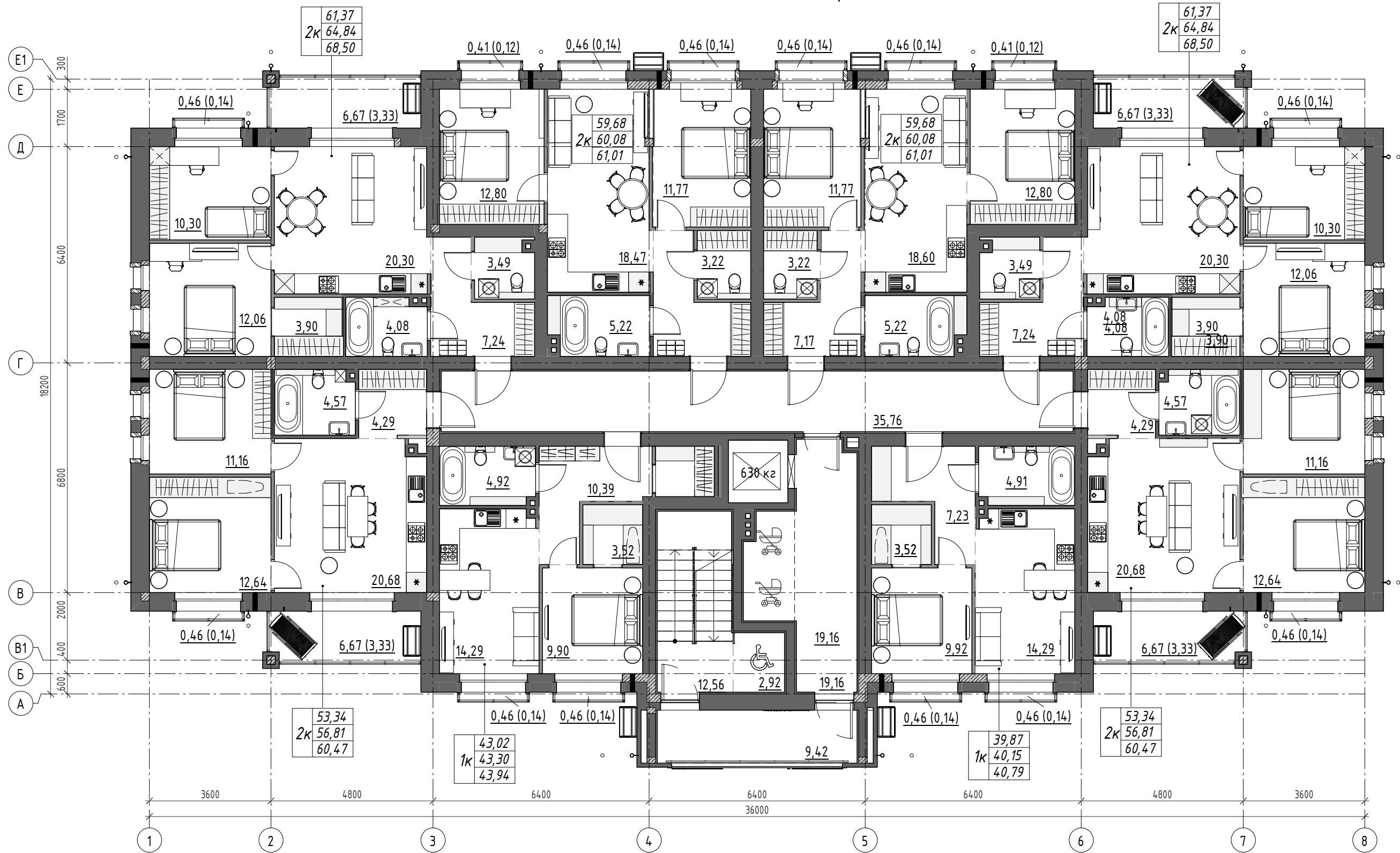
План 2 этажа на отм. +3,000
