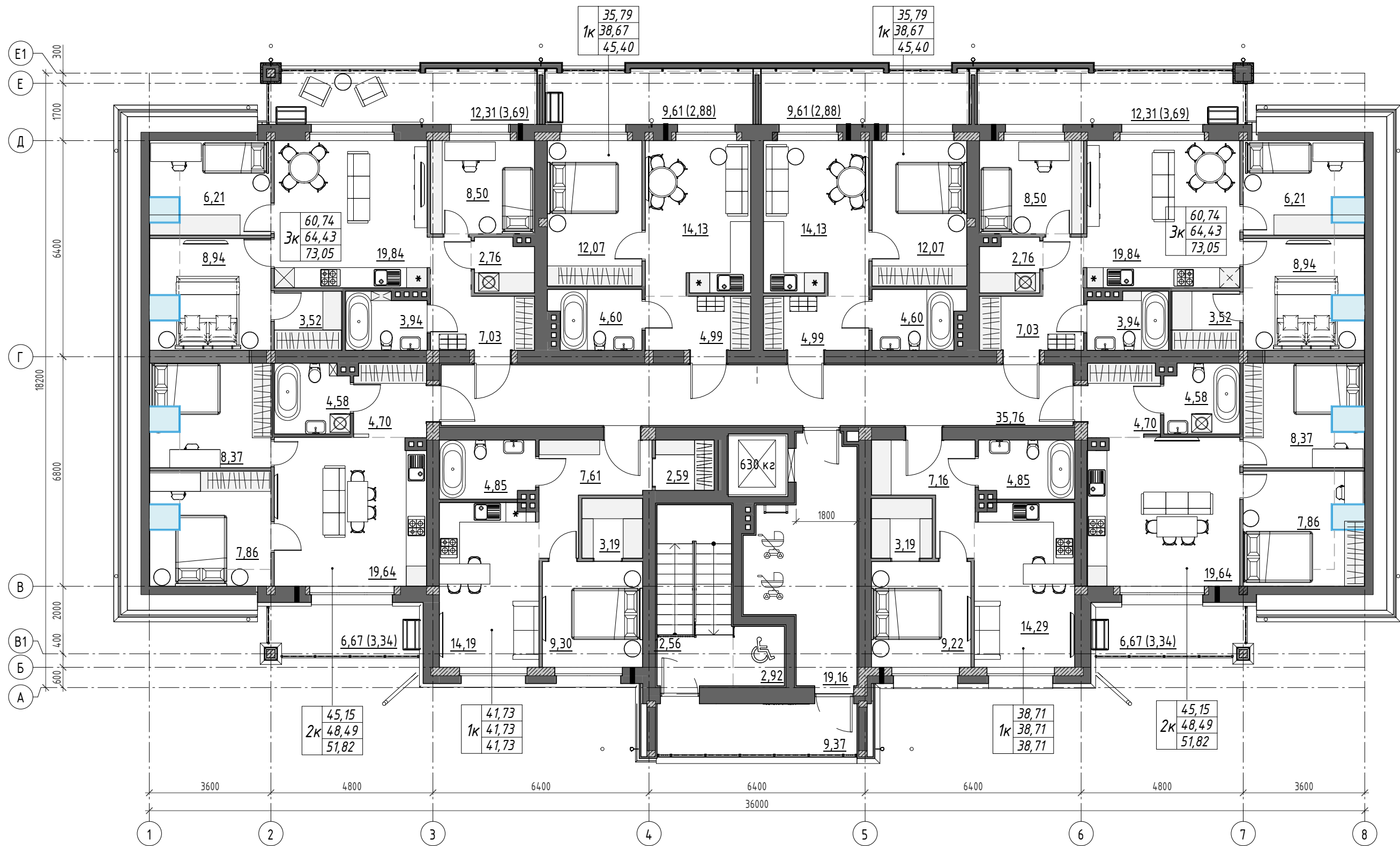
План 3 этажа на отм. +6,000
