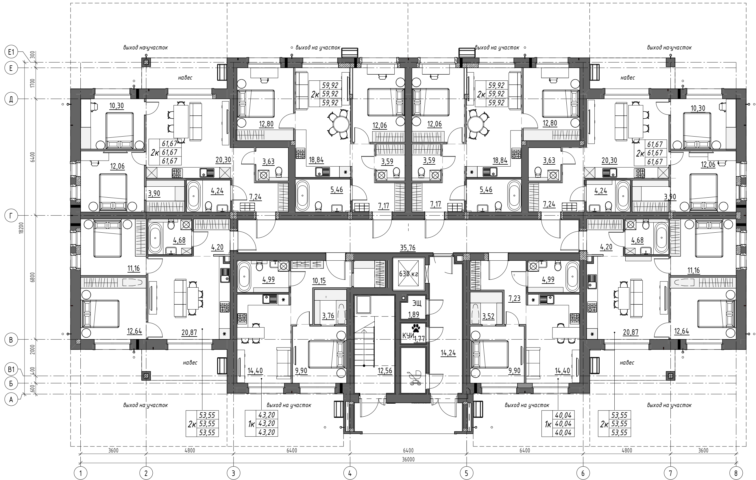
План 1 этажа на отм. 0,000
